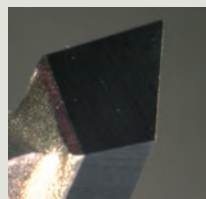
Nach 250 Schnitten in GENE0® Fensterprofilsystemen zeigt der Sägezahn eine äußerst geringe Abnutzung
